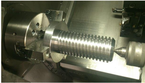
社内で製作した工具を使って のNC旋盤による台形ネジ加工
